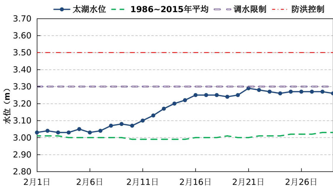
图2 2月太湖水位(8时)过程线
