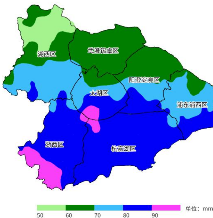
图1 2月太湖流域降水量等值面
