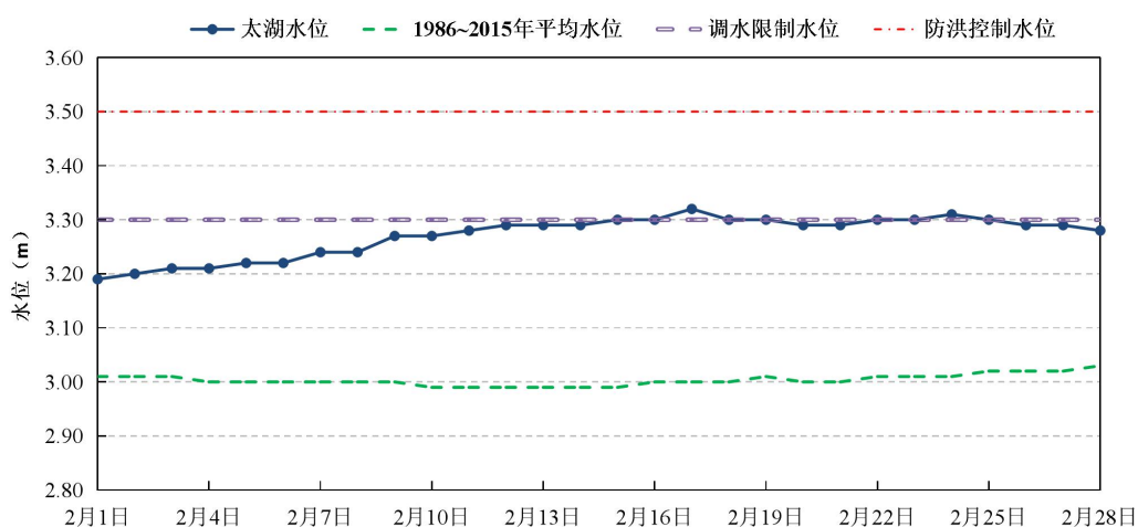
图2 2月太湖水位（8时）过程线
