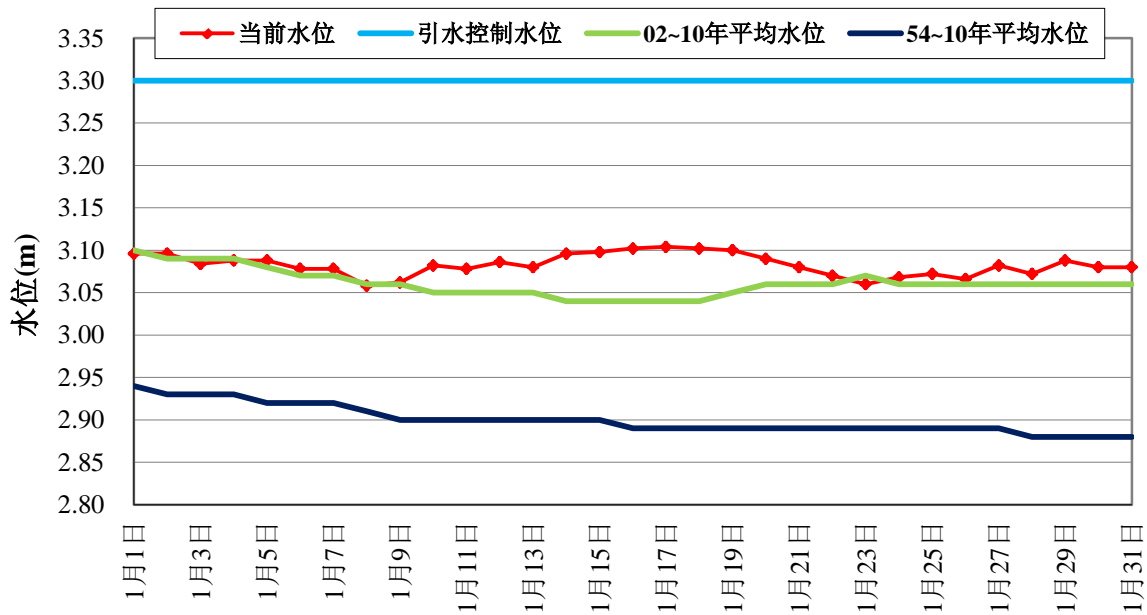
图 2 2015 年 1 月份太湖水位过程线图
