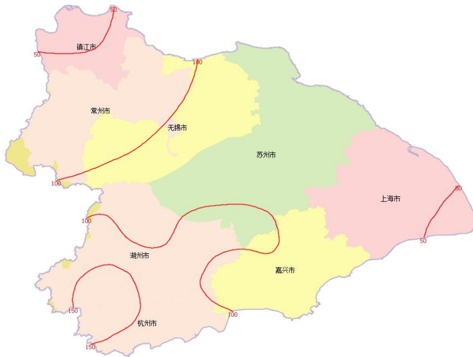
图 1 2018 年 4 月太湖流域降雨量等值线图
