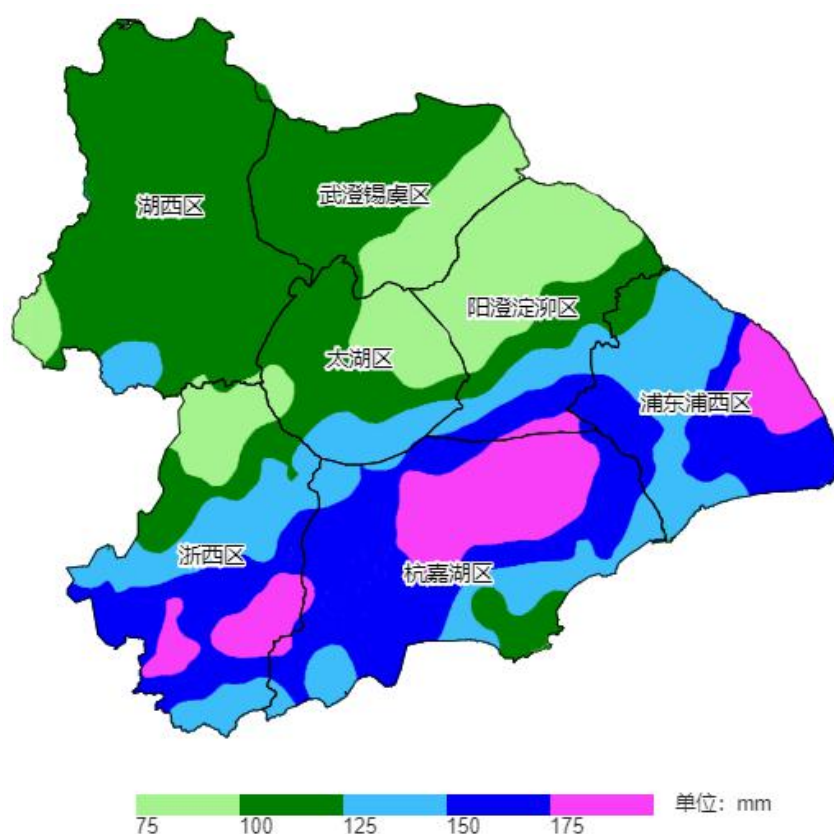
图 1 4 月太湖流域降水量等值面
