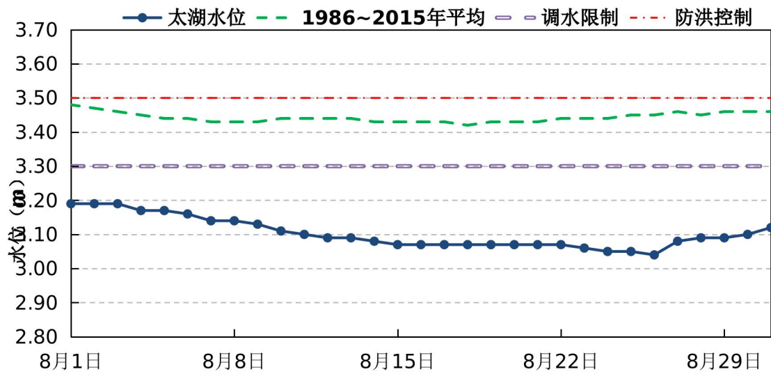
图2 8月太湖水位(8时)过程线
