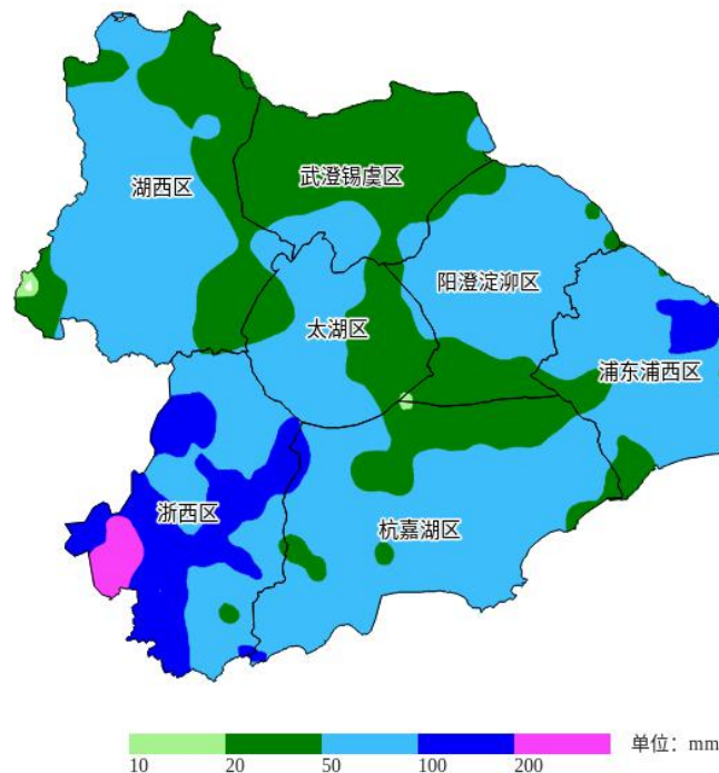
图 1 8 月太湖流域降水量等值面
