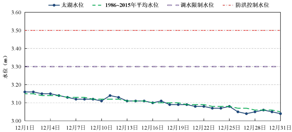
图2 12月太湖水位(8时)过程线
