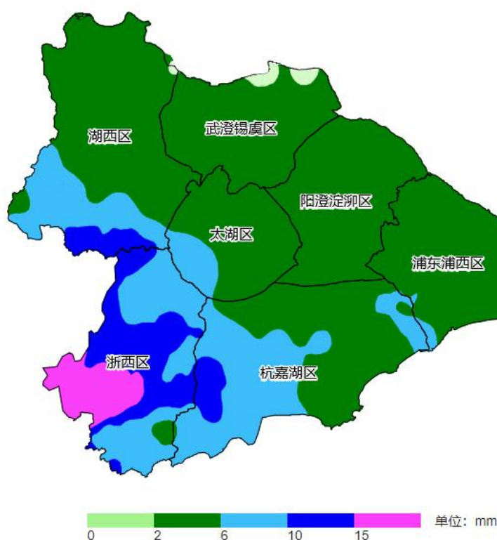
图 1 12 月太湖流域降水量等值面
