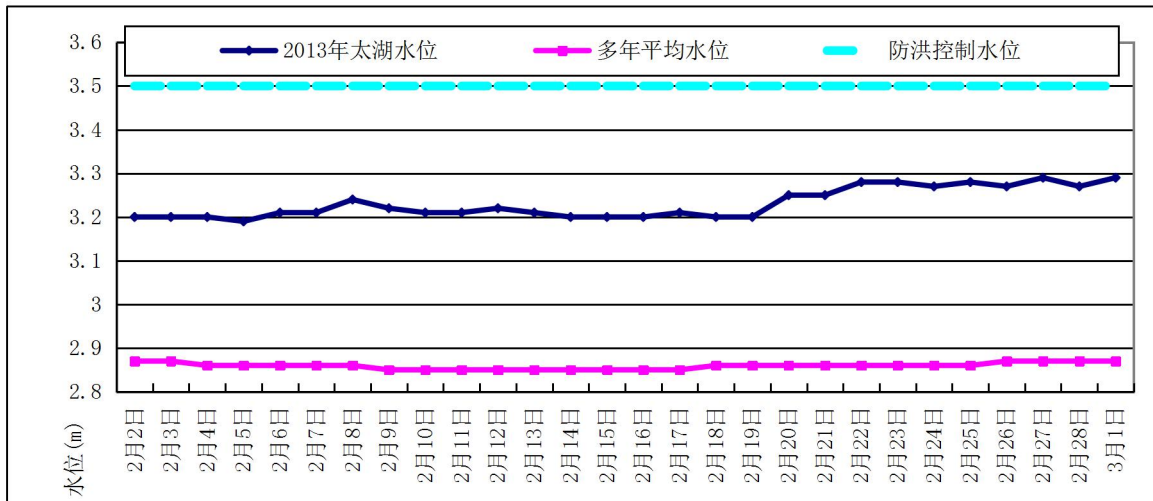
图2 2月份太湖水位过程线图
