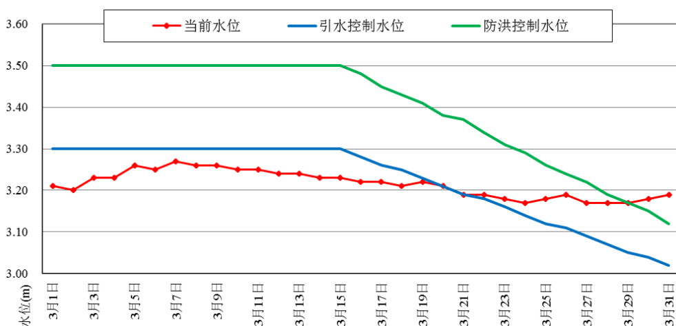
图2 3月份太湖水位过程线图
