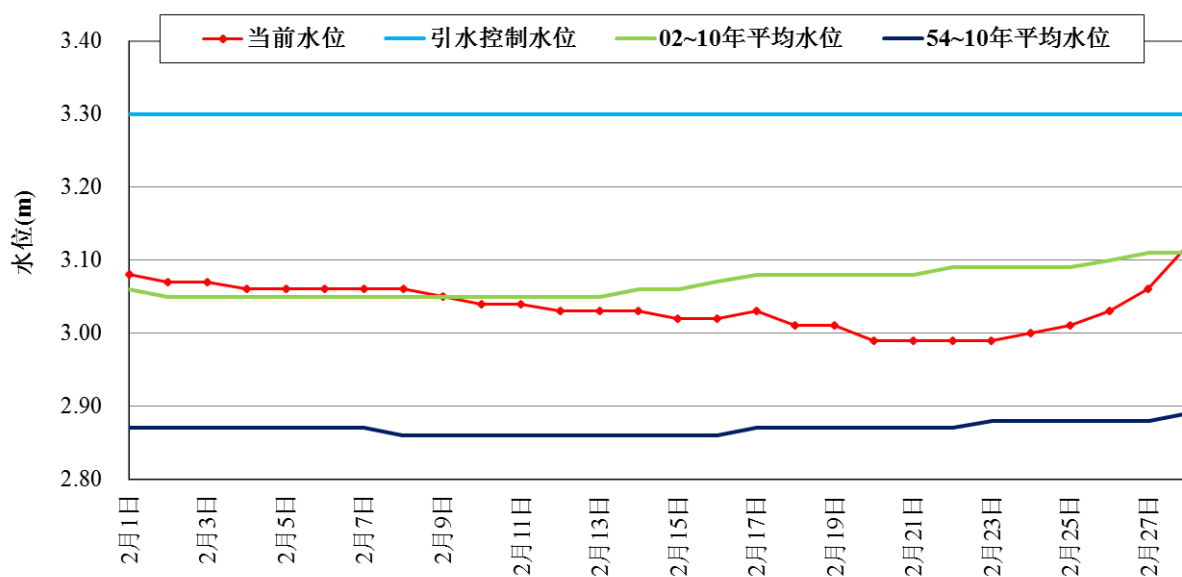
图 2 2015 年 2 月份太湖水位过程线图
